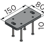
Platine + 4 vis TF 6.3x70 jusqu'à 1800 mm
