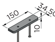
Demi-platine + 2 vis TF 6.3x70 jusqu'à 1800 mm
